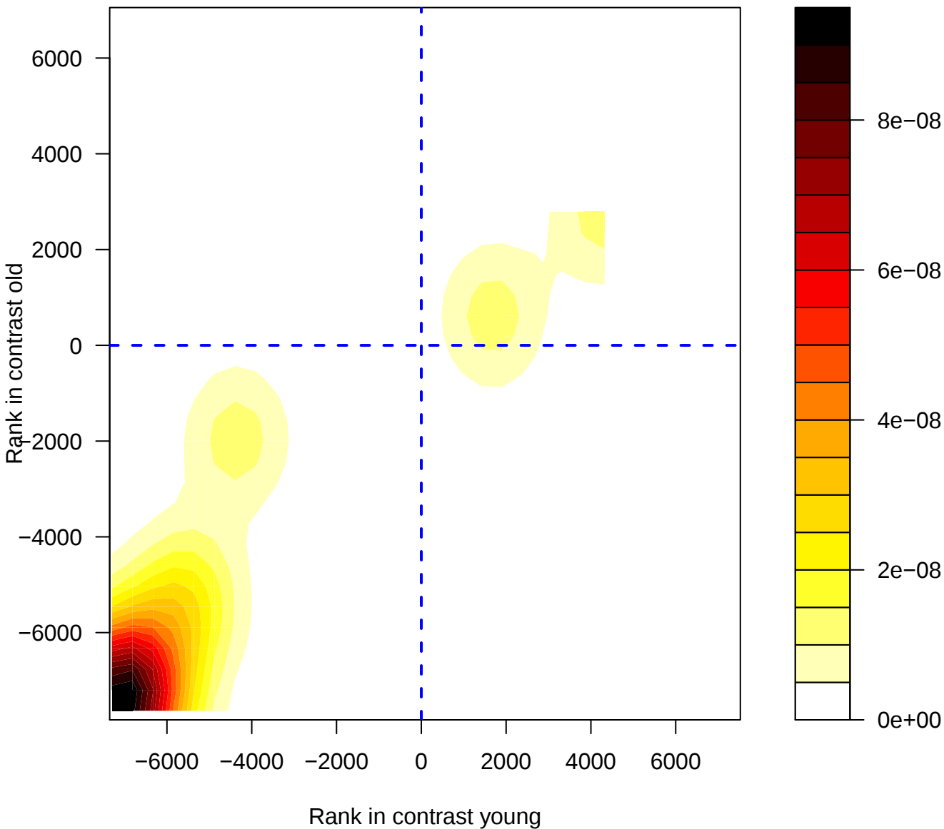
IRF8_None_None_72984
