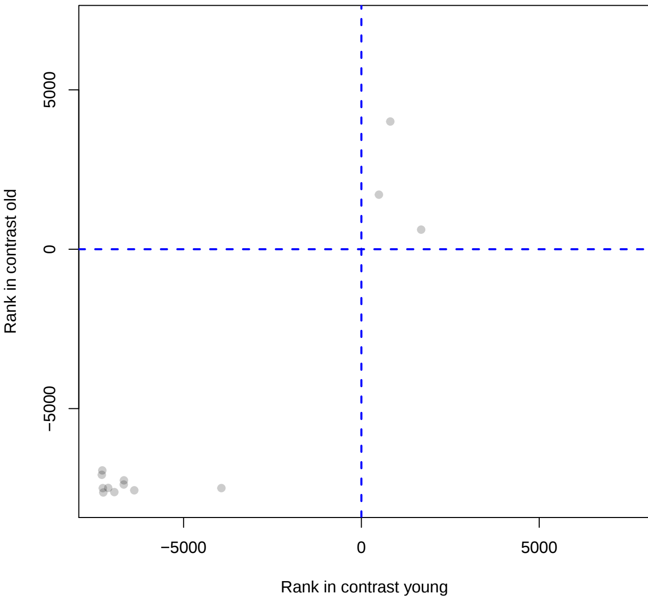
RPA_None_None_40211
