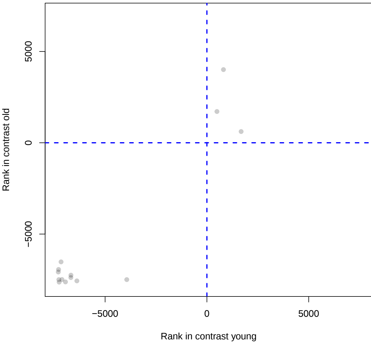
LMNB1_B1NIH_None_83601
