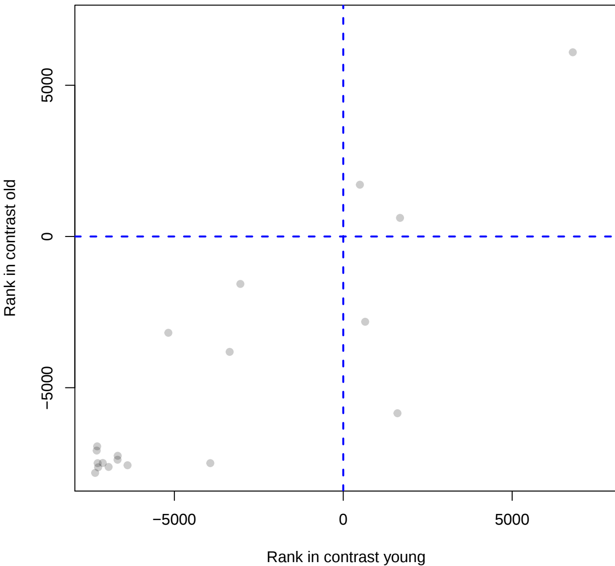
KMT2A_None_None_69455
