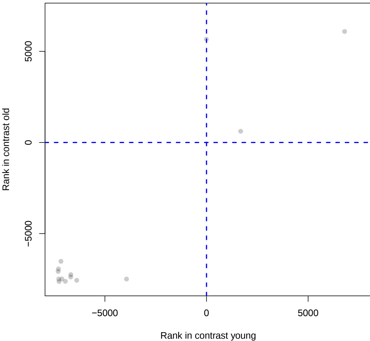
RB_None_EmbryonicFibroblast_71831
