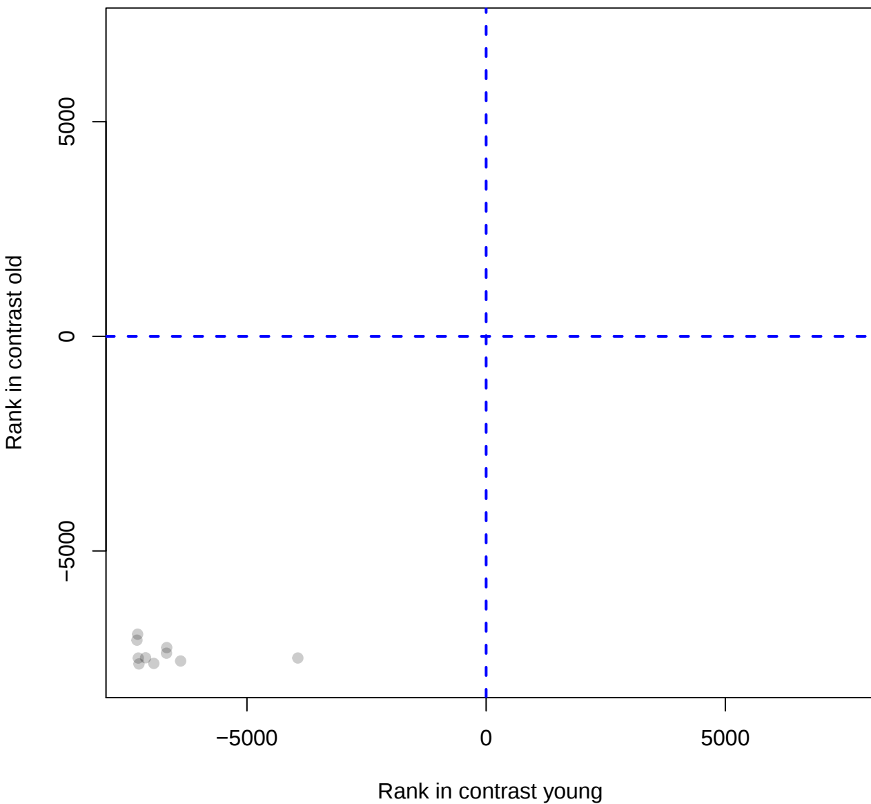
TOP2B_None_Neuron_53388
