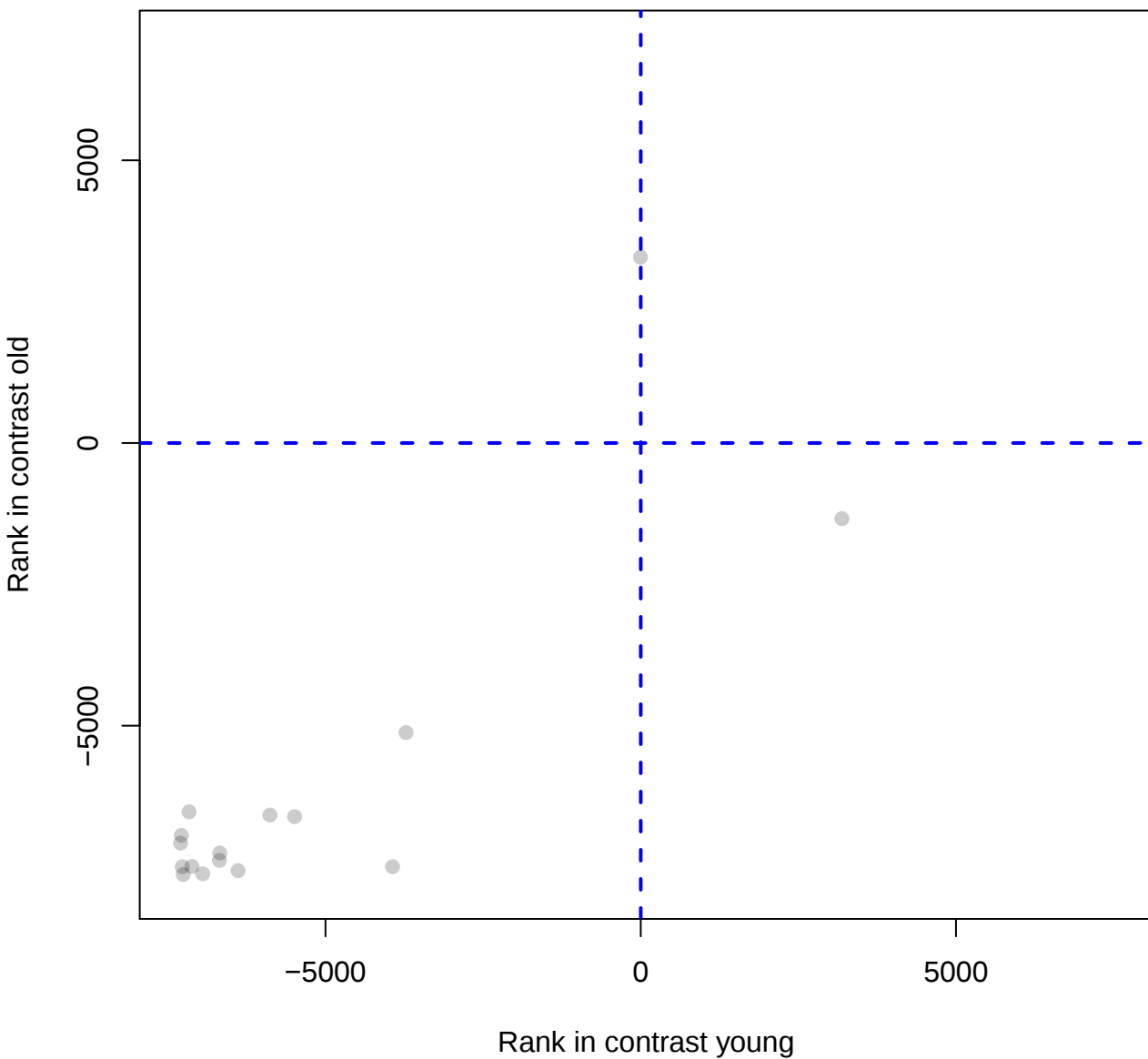
CDYL_None_None_85786
