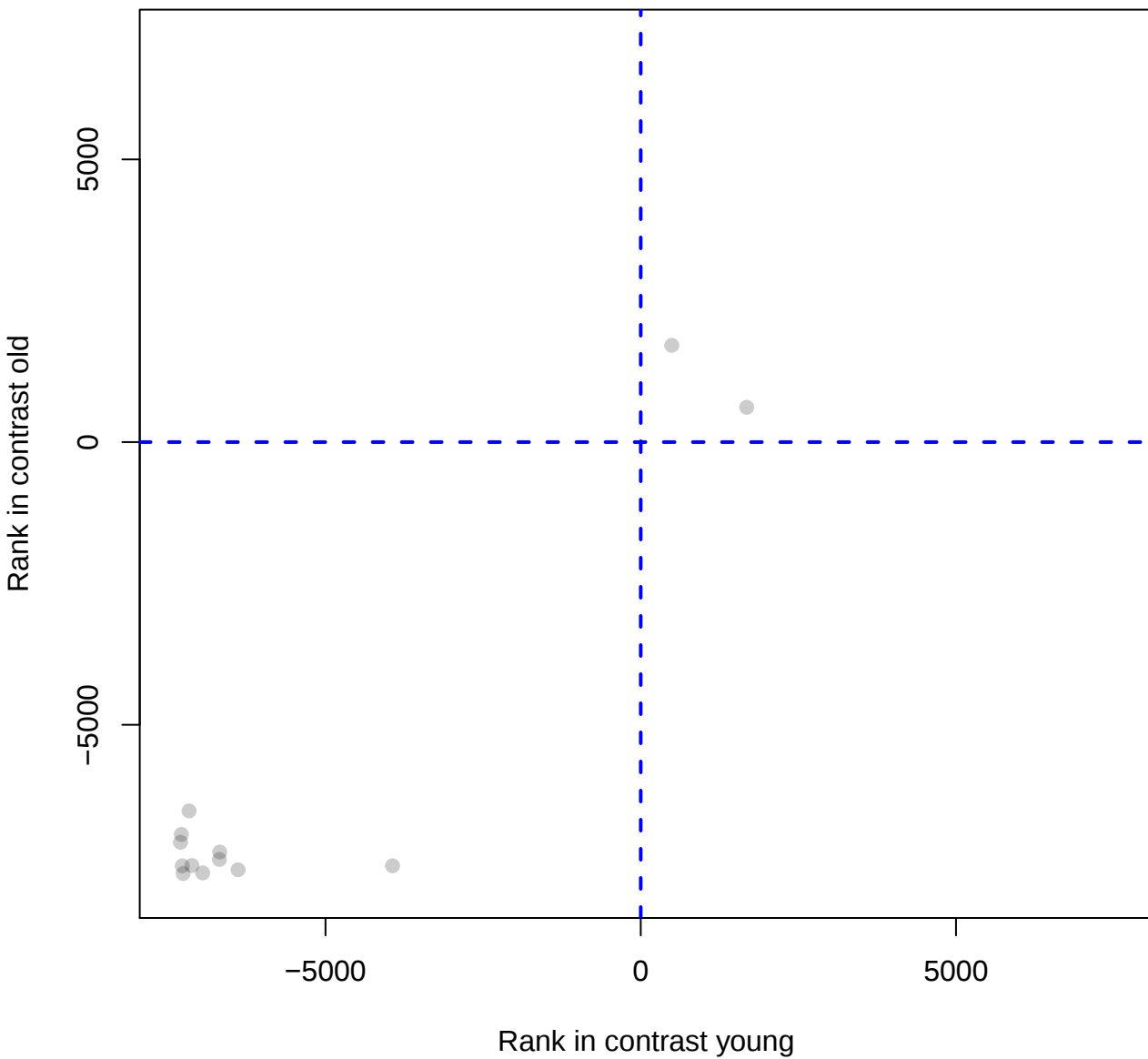
EZH1_None_None_88262
