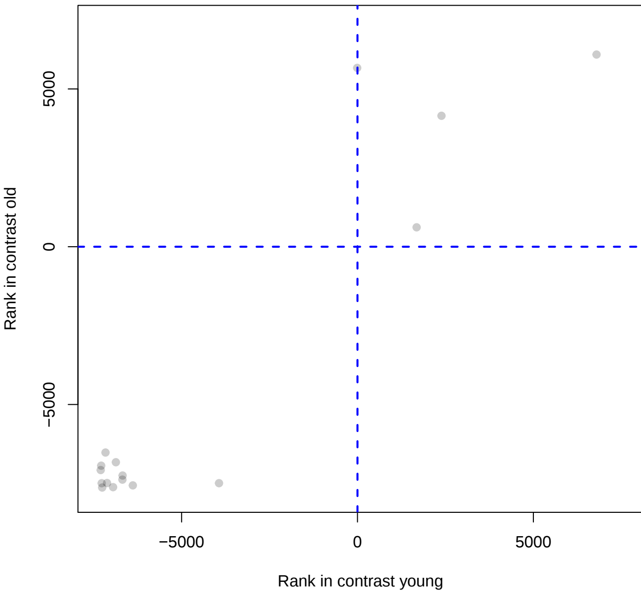
ESR1_None_None_69405
