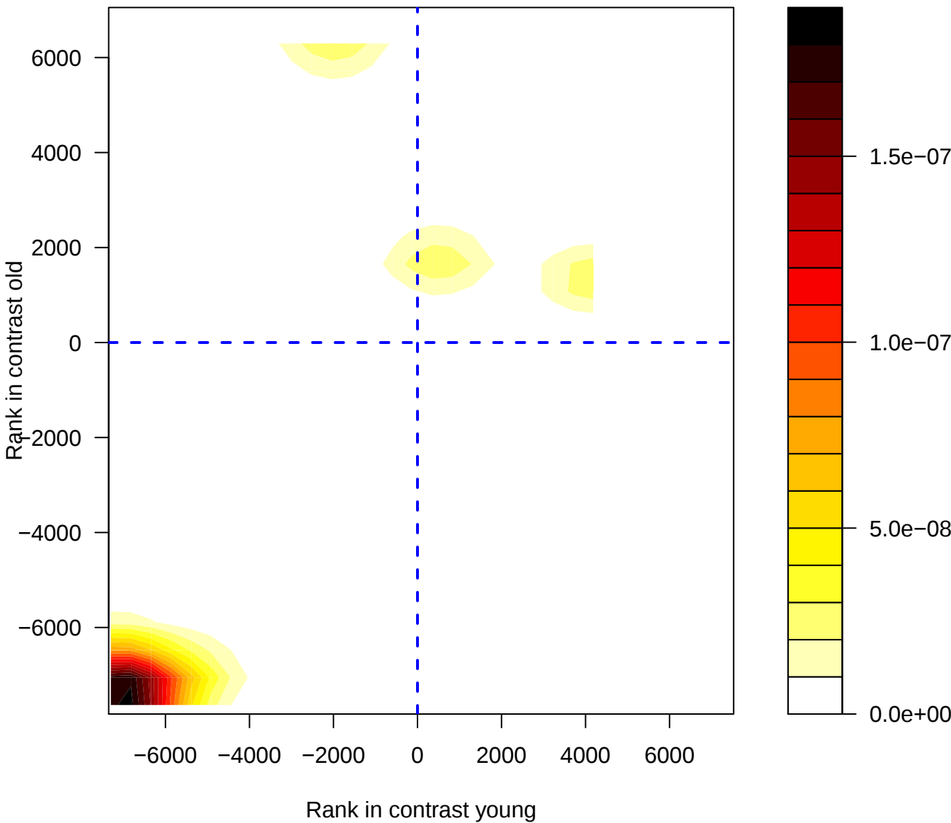
MTF2_None_EmbryonicStemCell_4392
