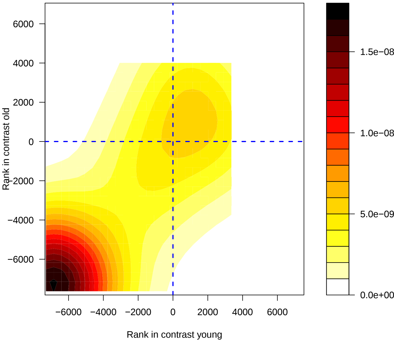
BAZ1B_None_None_70020
