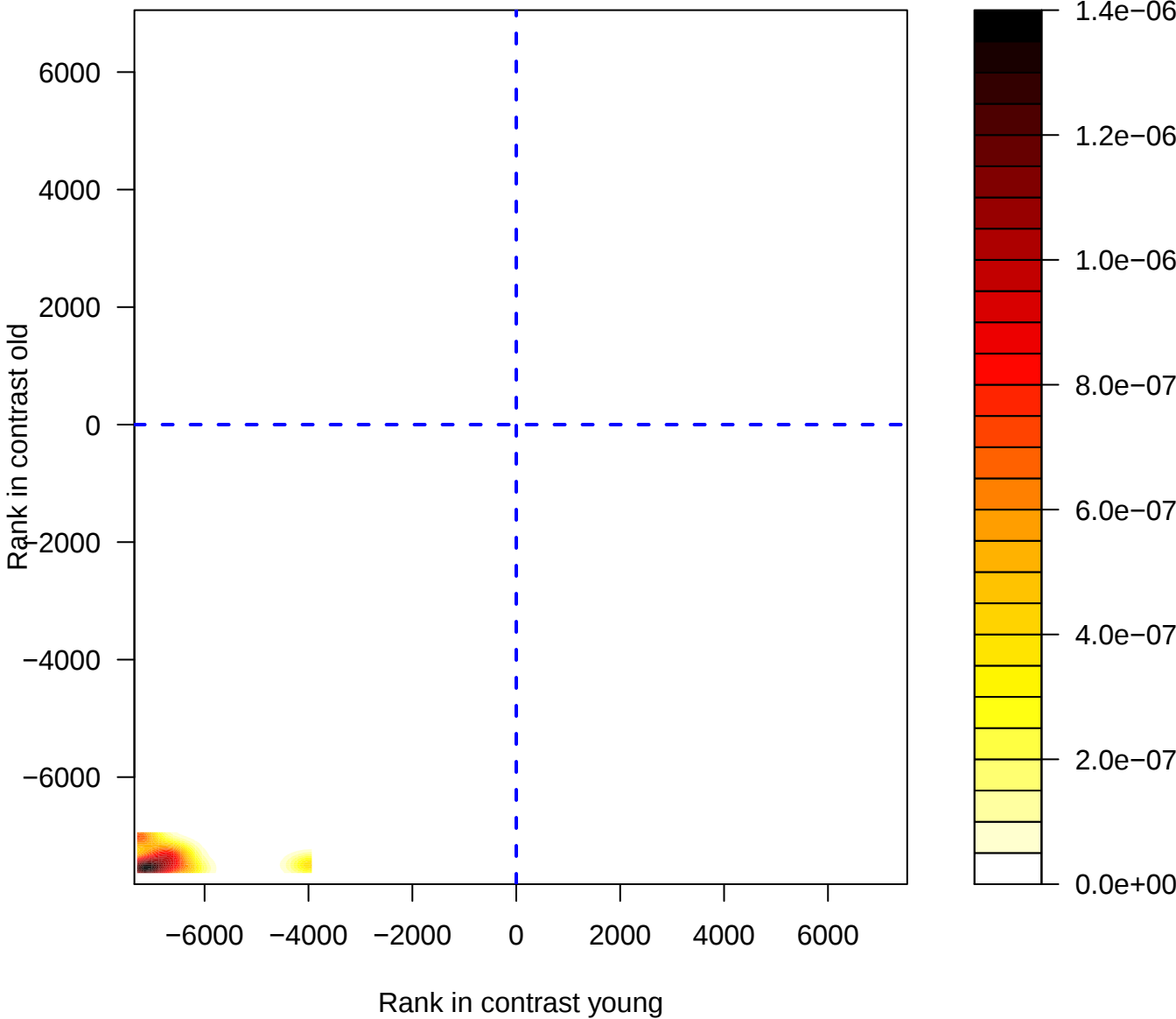
TOP2B_None_Neuron_53388
