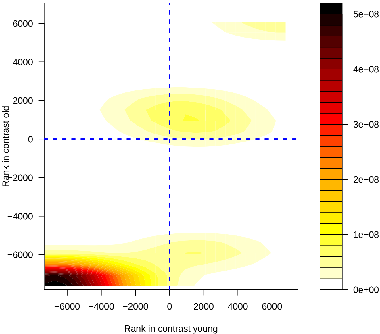
EP300_None_Stemcell_57746
