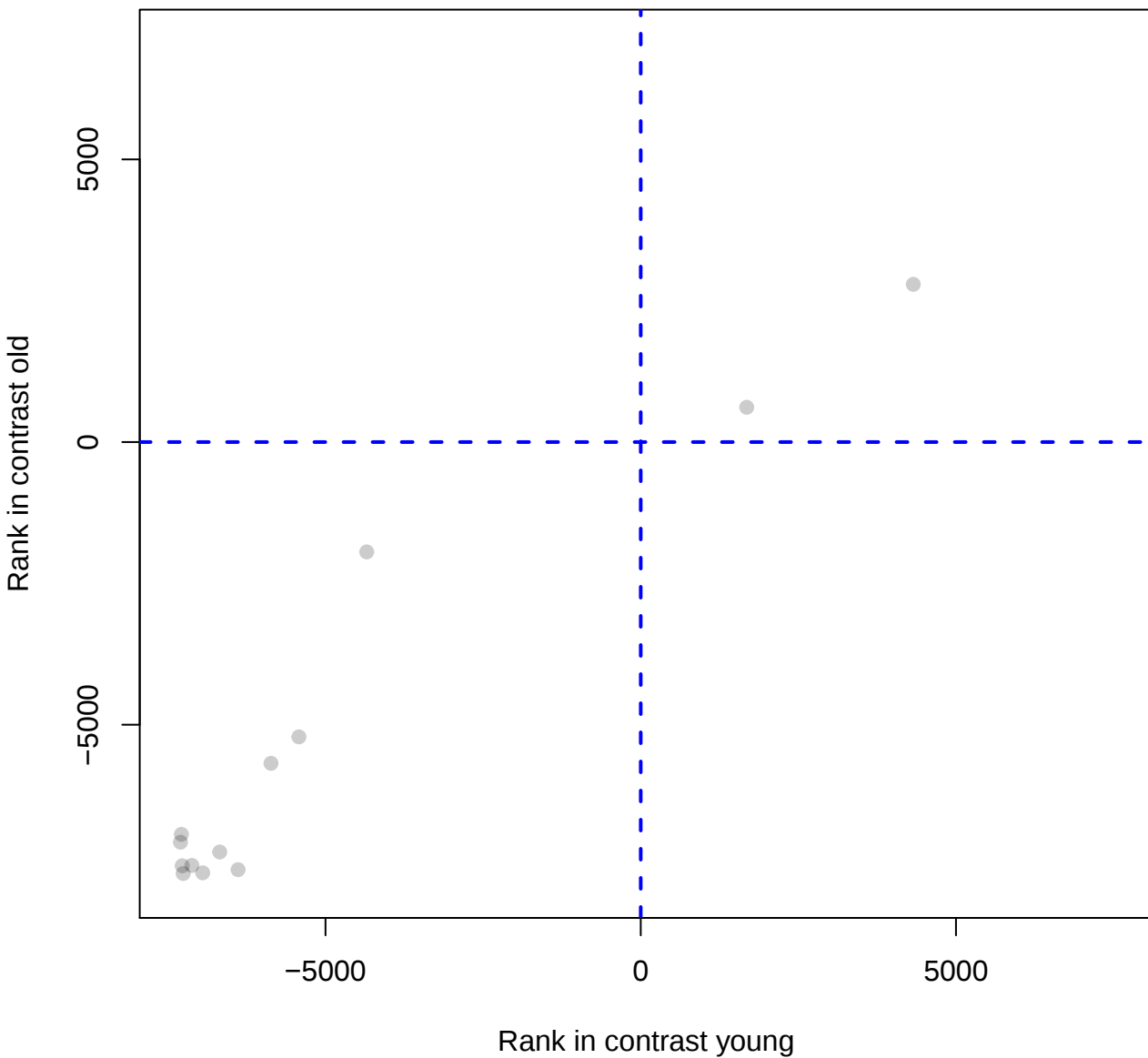
IRF8_None_None_72984
