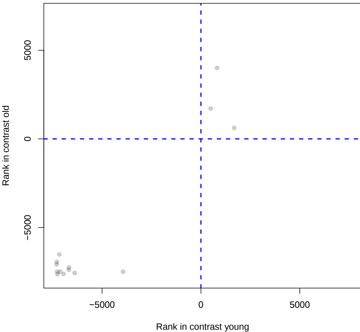
SIRT6_None_EmbryonicStemCell_52819
